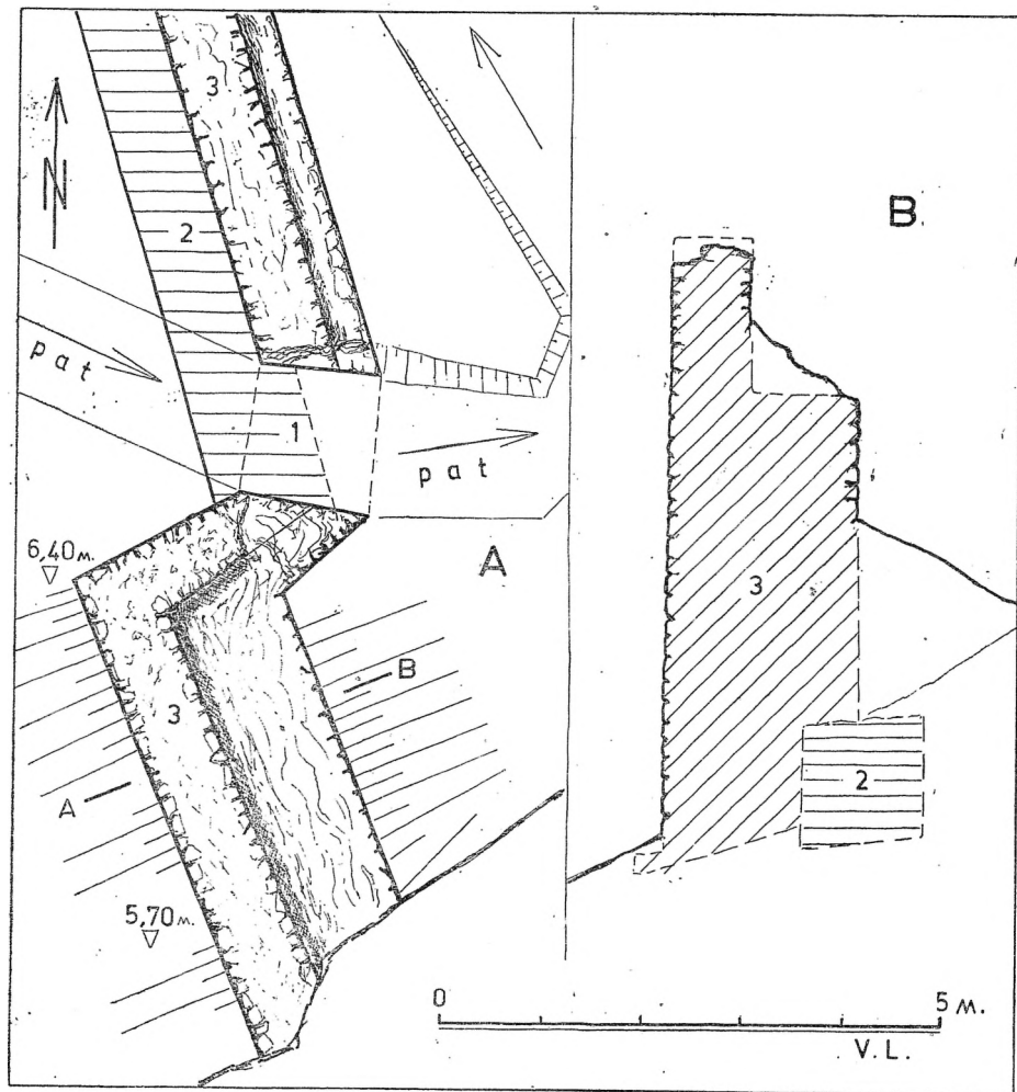
Сл. 4. Одбранбен бедем со влез во градот. План и пресек.
