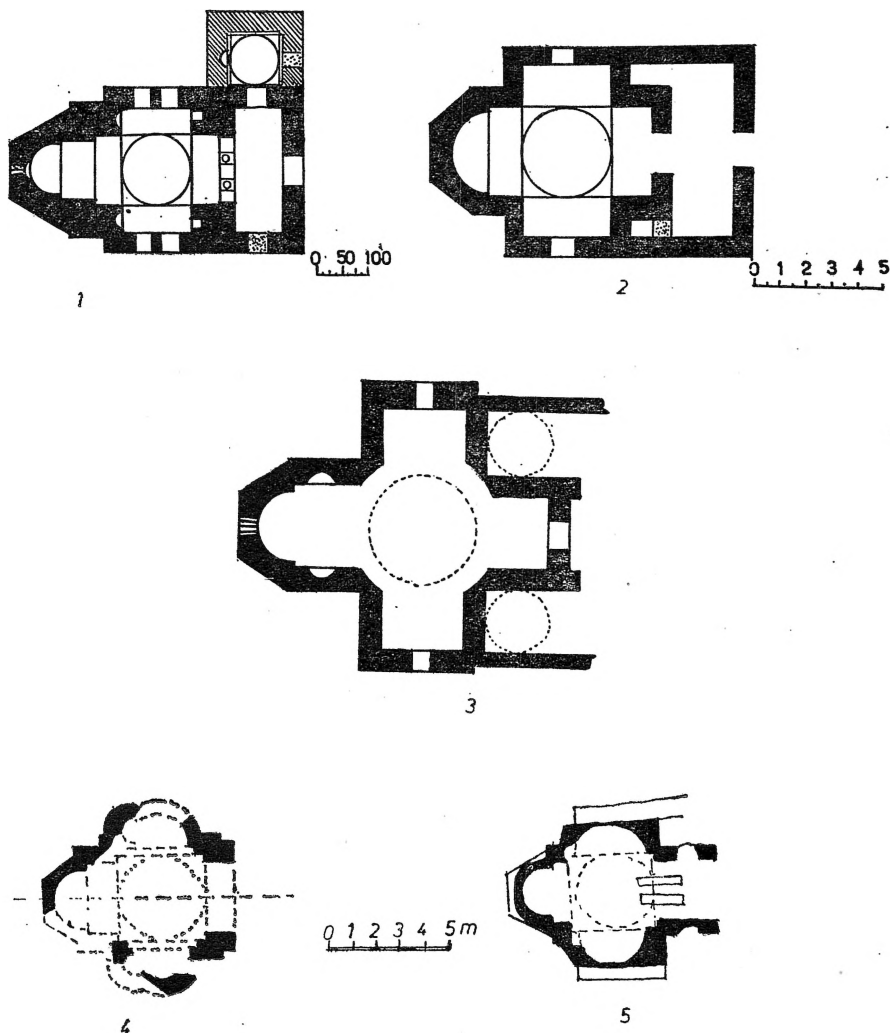
Сл. 1. Црквата Св. Ѓорѓи, Горен Козјак; Сл. 2. Црквата во Мородвиз; Сл. 3. Црквата Палеопанагија во Манолада. Според Ст. Михајлов, цртеж Арх. В. Миладинова; Сл. 4. Црквата на Св. Климент, Охрид; Сл. 5. Црквата на Св. Наум, Охридско Езеро. Според Д. Коцо, цртеж Арх. Н. Ничота.
